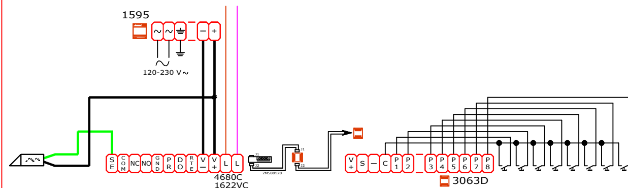
Externe beldrukkers
